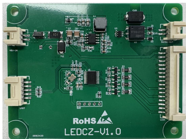
正面图
