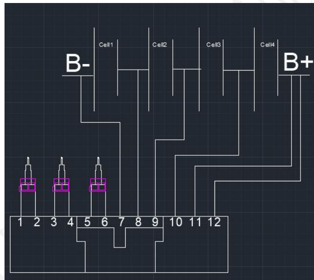
采样接口（12PIN 排插）
